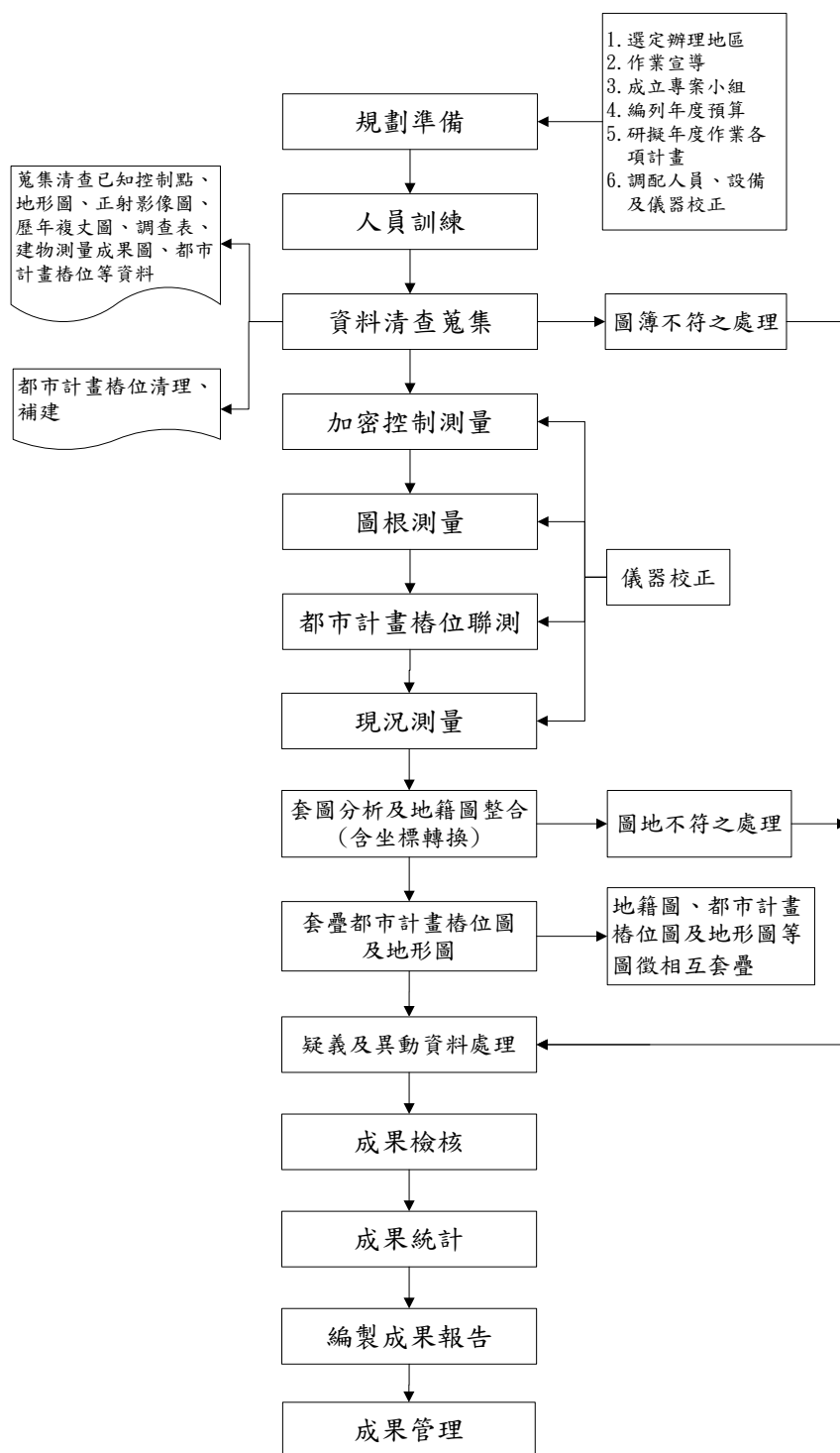
圖 2-1 作業流程圖
