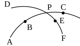
圖 9-6 圓弧與圓弧求交點
